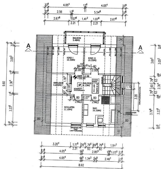
GRUNDRISS OBERGESCHOSS
