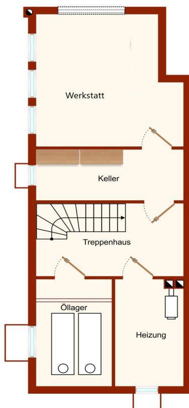
Kellergeschoss
