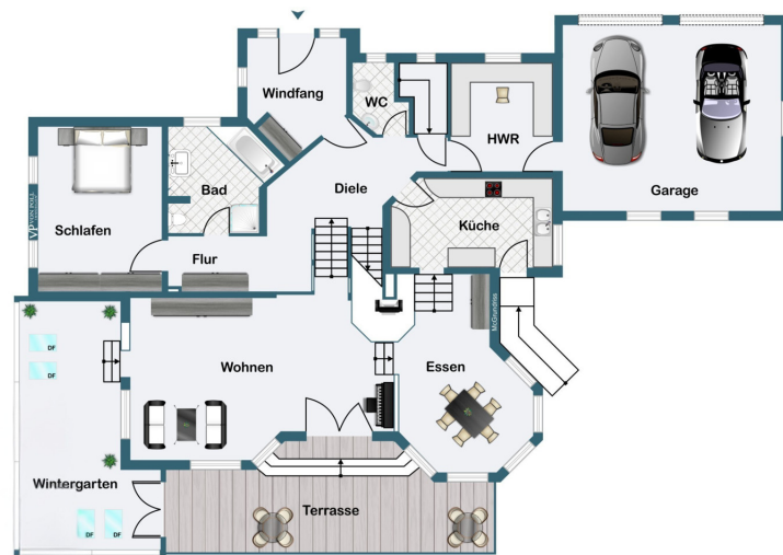
Erdgeschoss
