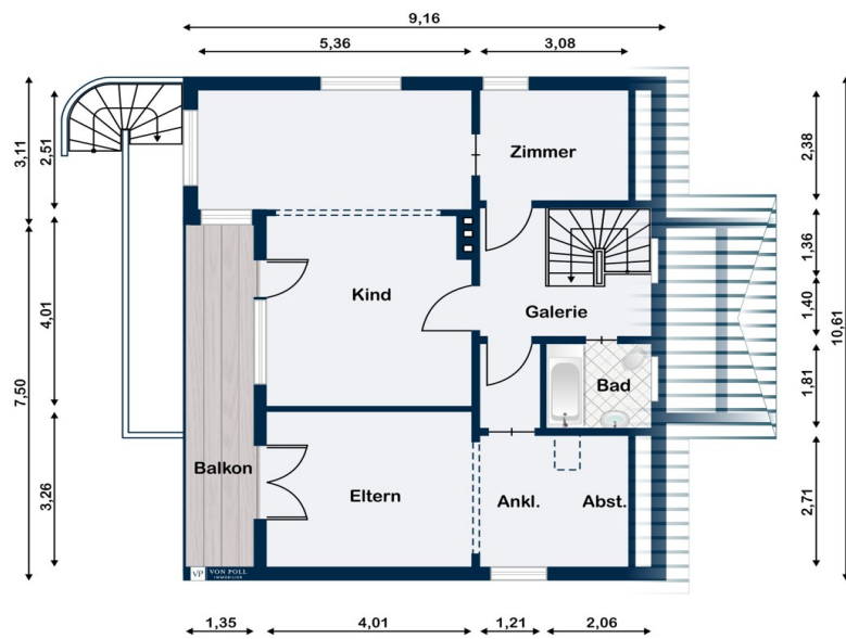
Dachgeschoss
