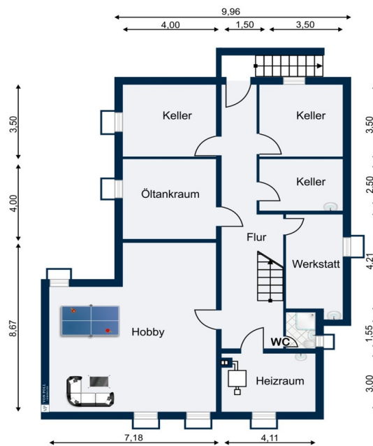
Kellergeschoss
