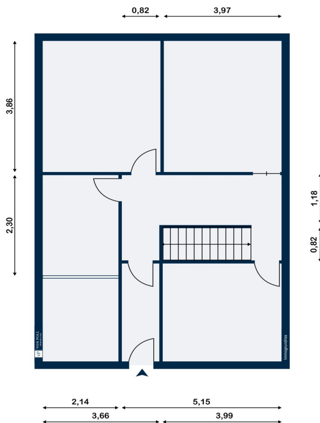
Kellergeschoss
