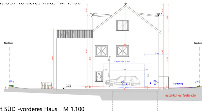
Ansicht OST - vorderes Haus M 1.100
