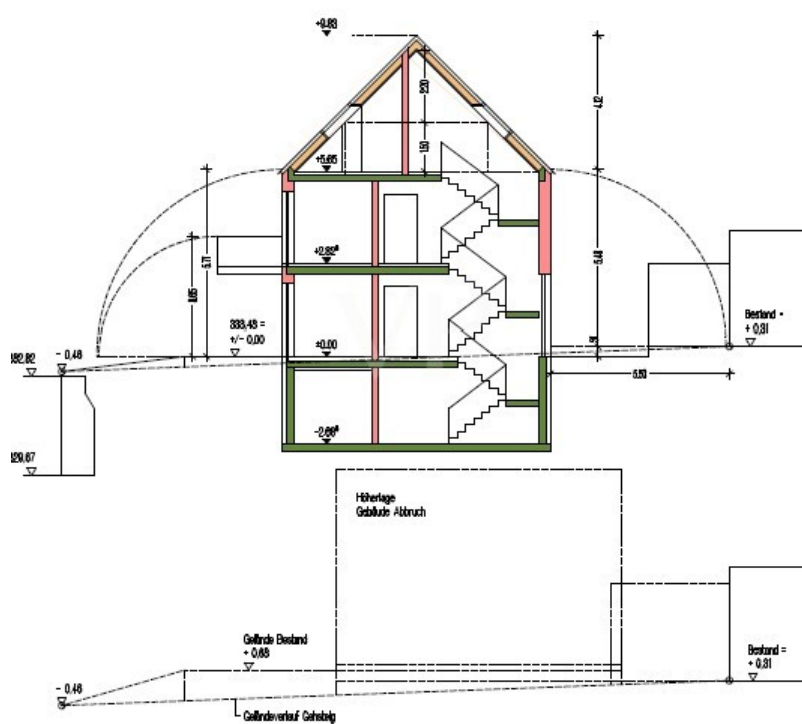
Schnitt A-A
