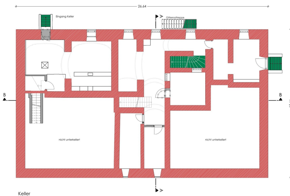
Keller
