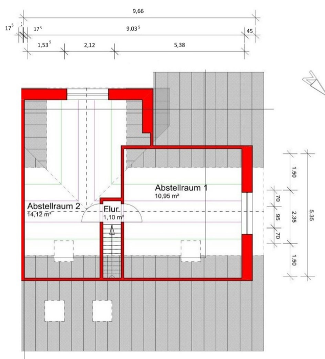
Grundriss Dachgeschoss
