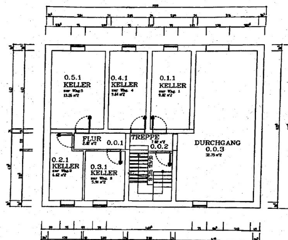
GRUNDRISS KELLERGESCHOSS M 1 : 100
