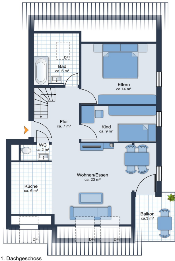
1. Dachgeschoss
