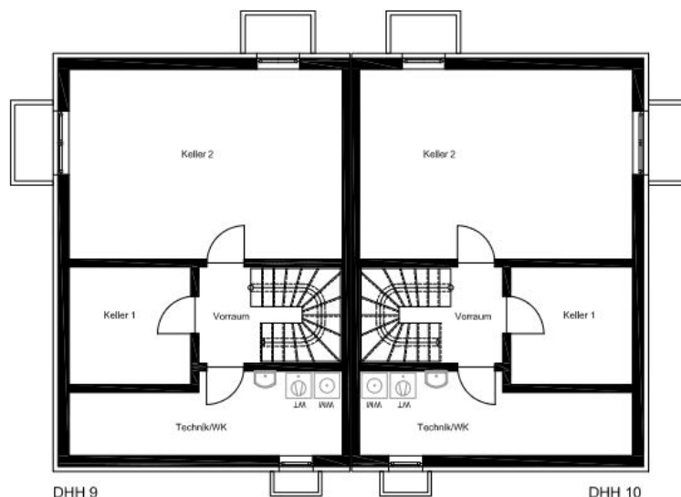
Grundriss UG
