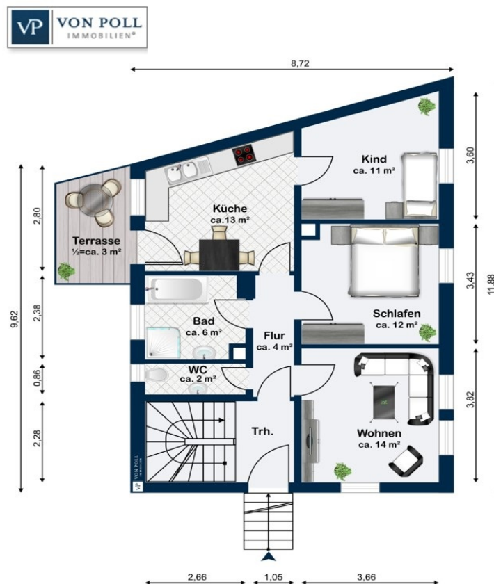
Erdgeschoss
