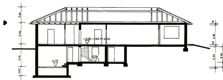
SCHNITT A-A
