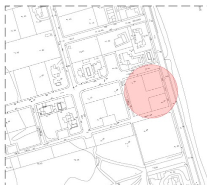
SITUACIÓN Escala 1:500
