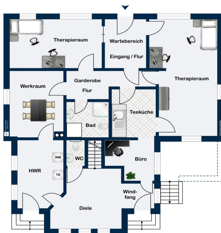
Erdgeschoss
