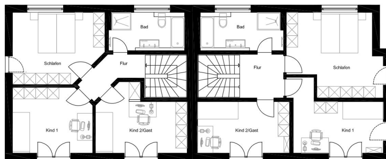
Grundriss OG
