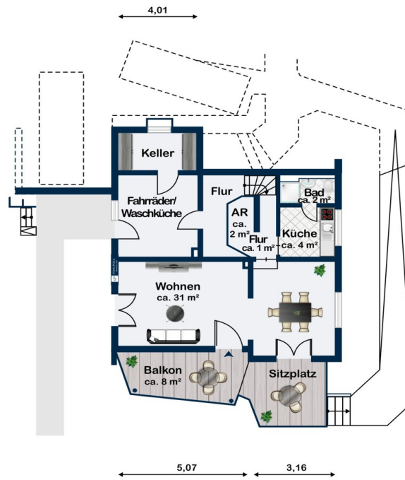
Untergeschoss
