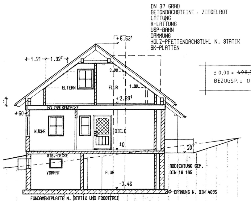
SCHNITT A-A
