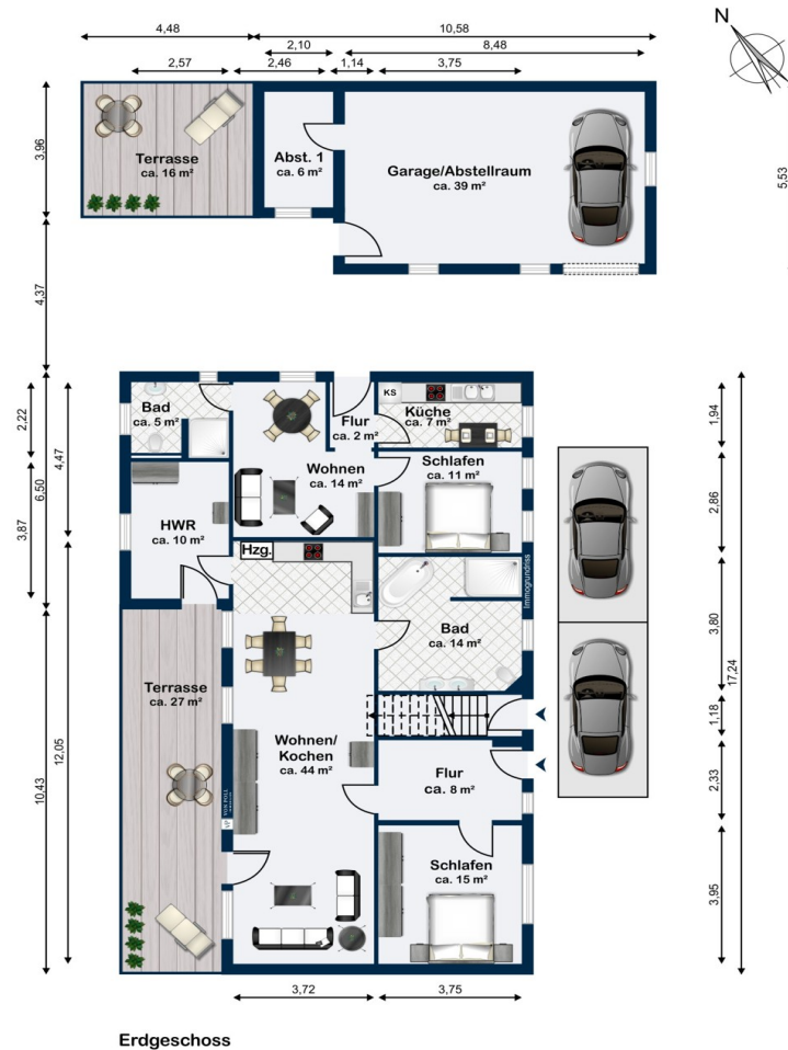
Erdgeschoss
