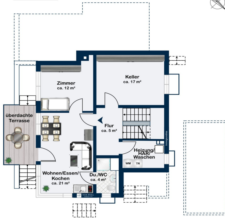
Kellergeschoss
