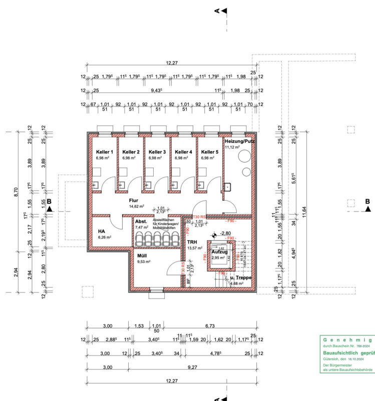
GRUNDRISS UG
