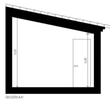
SECCIÓN A-A
