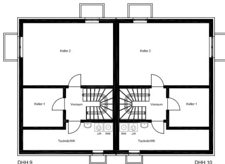
Grundriss UG
