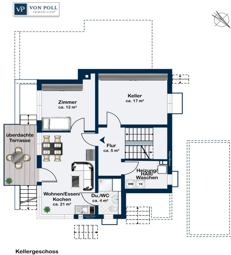
Kellergeschoss
