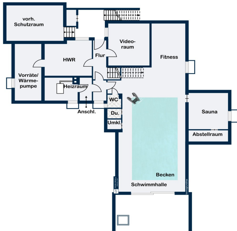
Untergeschoss
