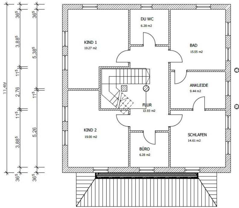
OBERGESCHOSS M 1 : 100
