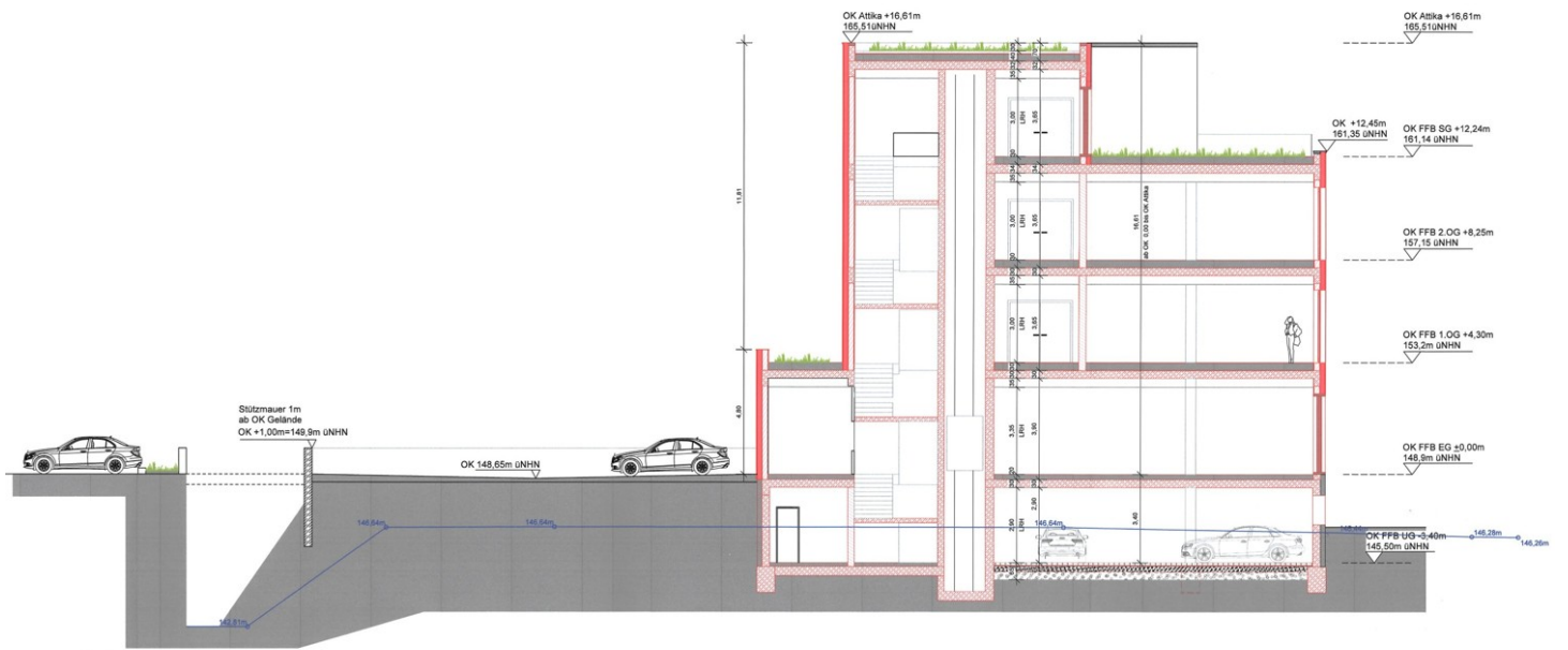
Schnitt C-C
