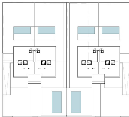
EMPLAZAMIENTO Escala 1:500
